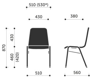
K43 / K44
